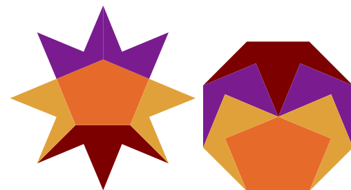
Razdelitev pentagrama v desetkotnik.
