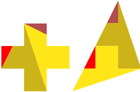
Razdelitev križa v trikotnik.
