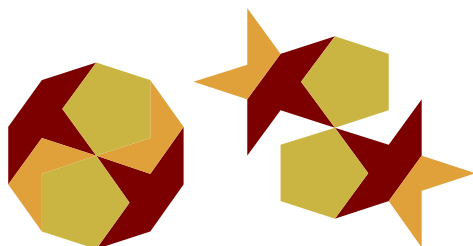
Razdelitev dvanajstograma v dva heksagrama (eden je izpuščen).
