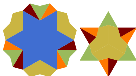
Razdelitev dvanajstograma v dva heksagrama (eden je izpuščen).
