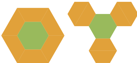
Razdelitev šestkotnika v štiri.
