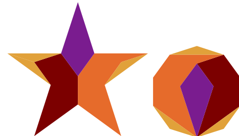
Razdelitev pentagrama v desetkotnik.
