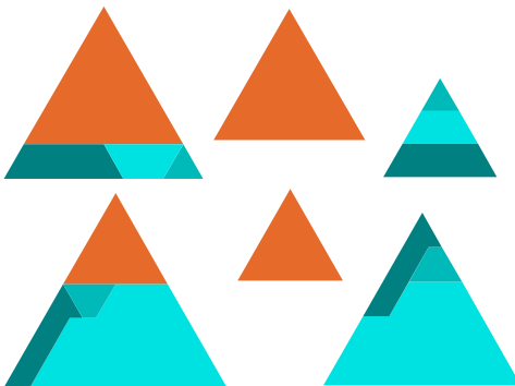
Razdelitev dveh trikotnikov v dva.
