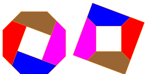
Bennettova razdelitev osemkotnika v kvadrat
